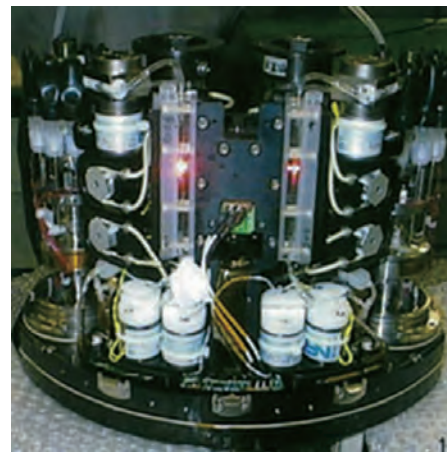
写真3 「宇宙滞在における生物時間：ゾウリムシのクローン寿命の変動」ミッションのための搭載実験装置試作品（千代田化工アドバンストソリューション提供）。
